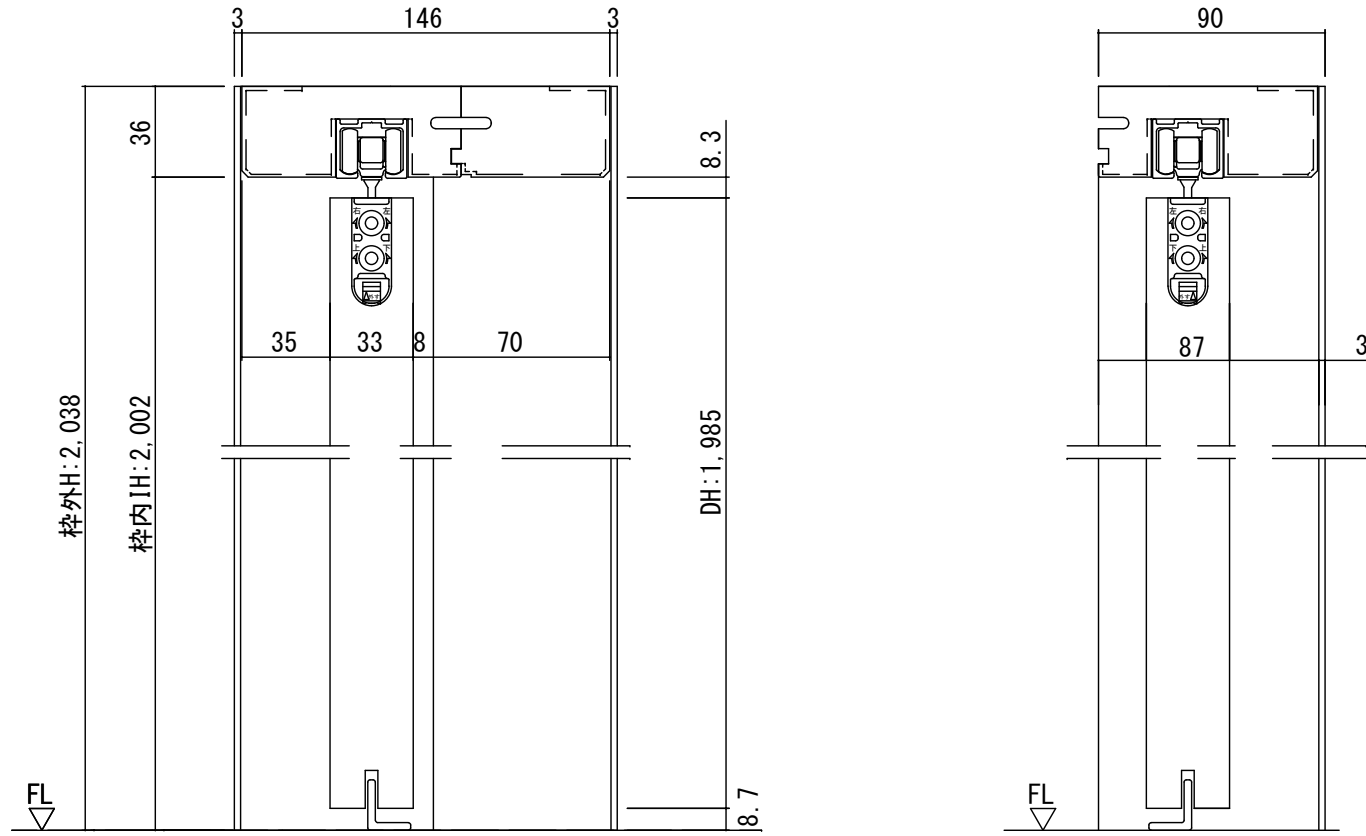
断面図
